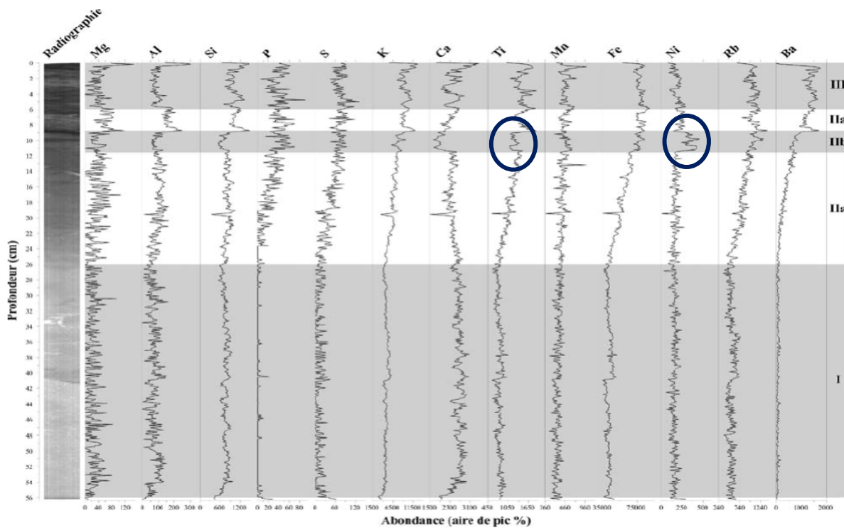
Figure 4. Radiographie et profils stratigraphiques d'éléments chimiques sélectionnés
