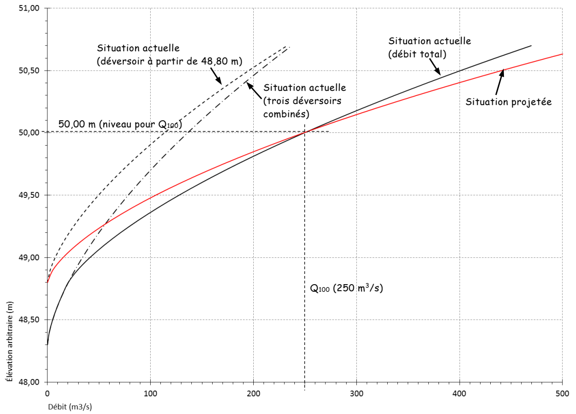
Figure 2 Capacité transitoire du déversoir en enrochement du barrage Étang Stater (situation actuelle et projetée).
